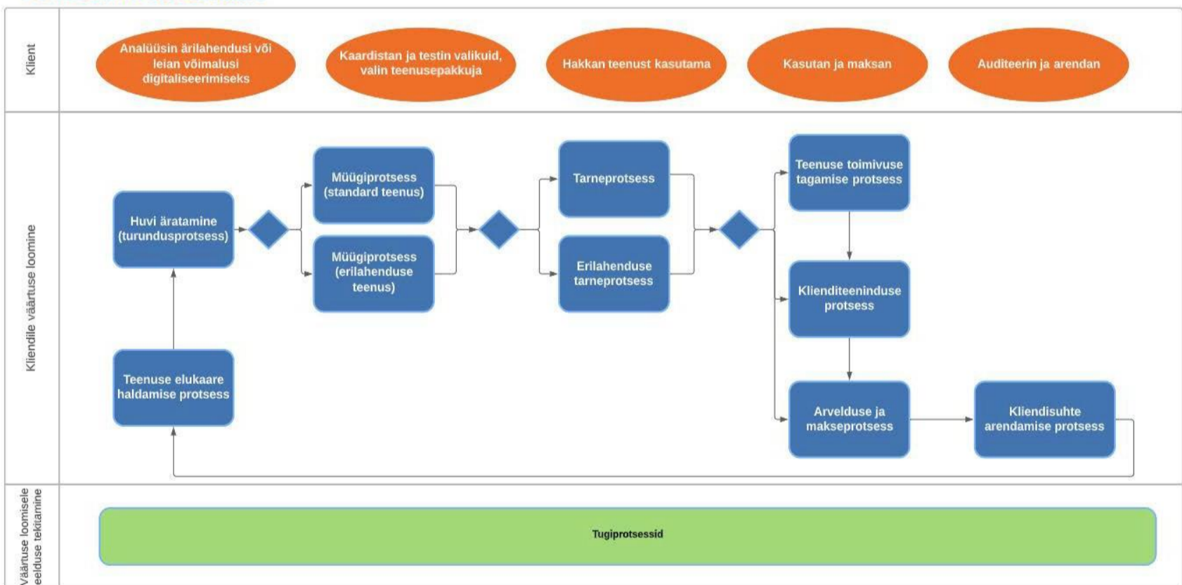
Ärikliendi Protsessikaart
